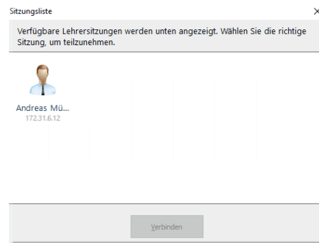
Abbildung 17: Sitzungsliste
