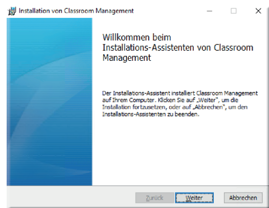
Abbildung 5: Installations-Assistent
