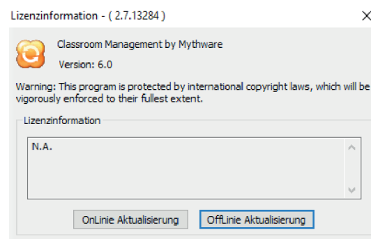
Abbildung 19: Lizenzinformation
