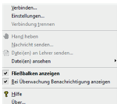
Abbildung 18: Taskleiste
