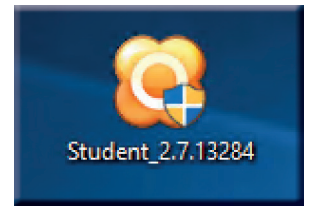
Abbildung 1: Installationsdatei Schüler
