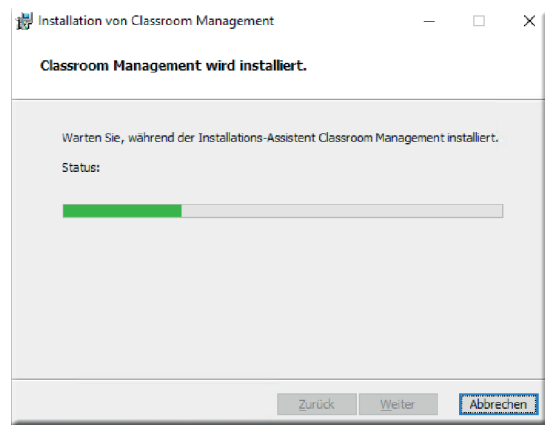
Abbildung 12: Installationsvorgang - Warten
